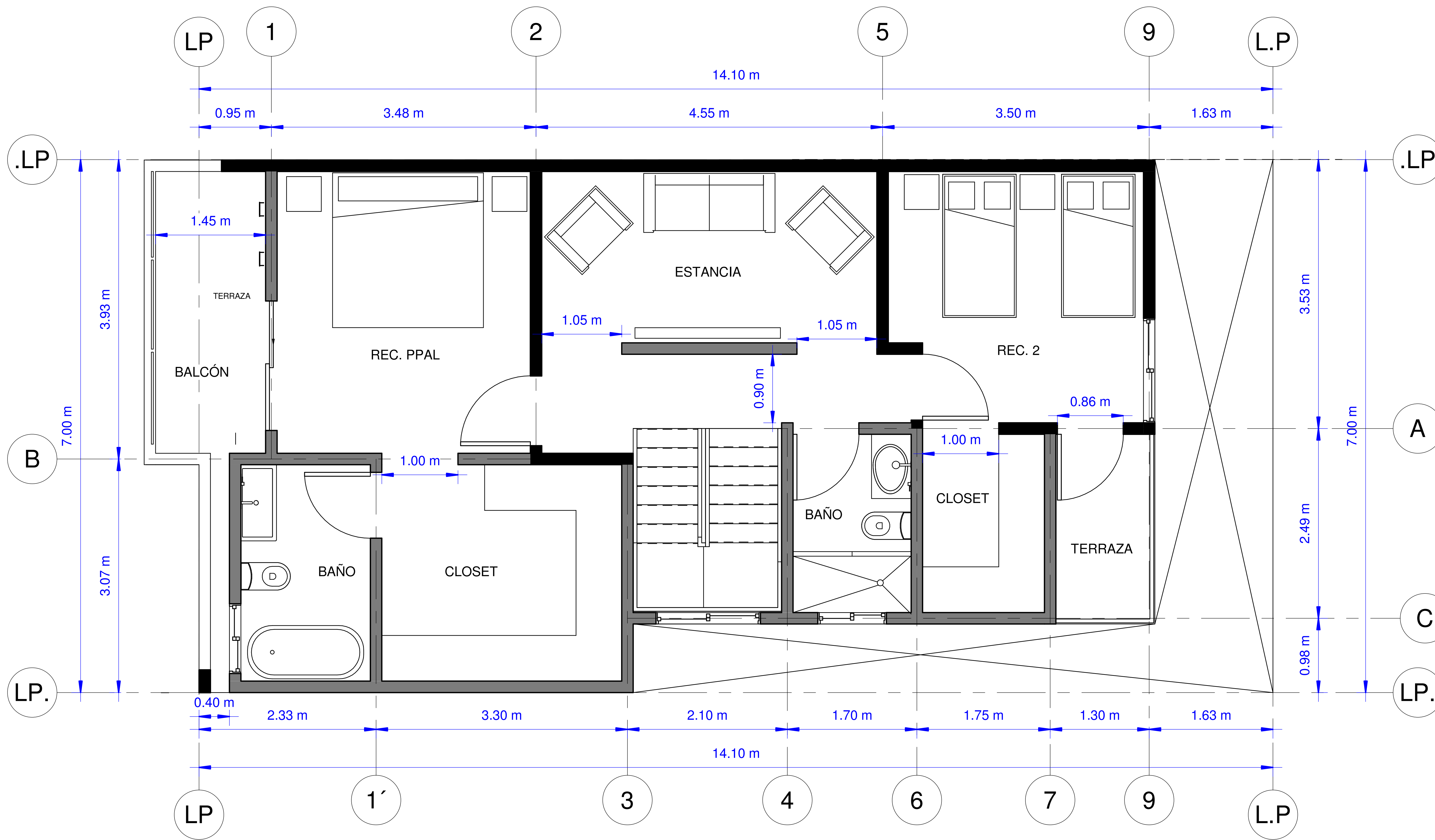
PLANTA ARQUITECTONICA ALTA
