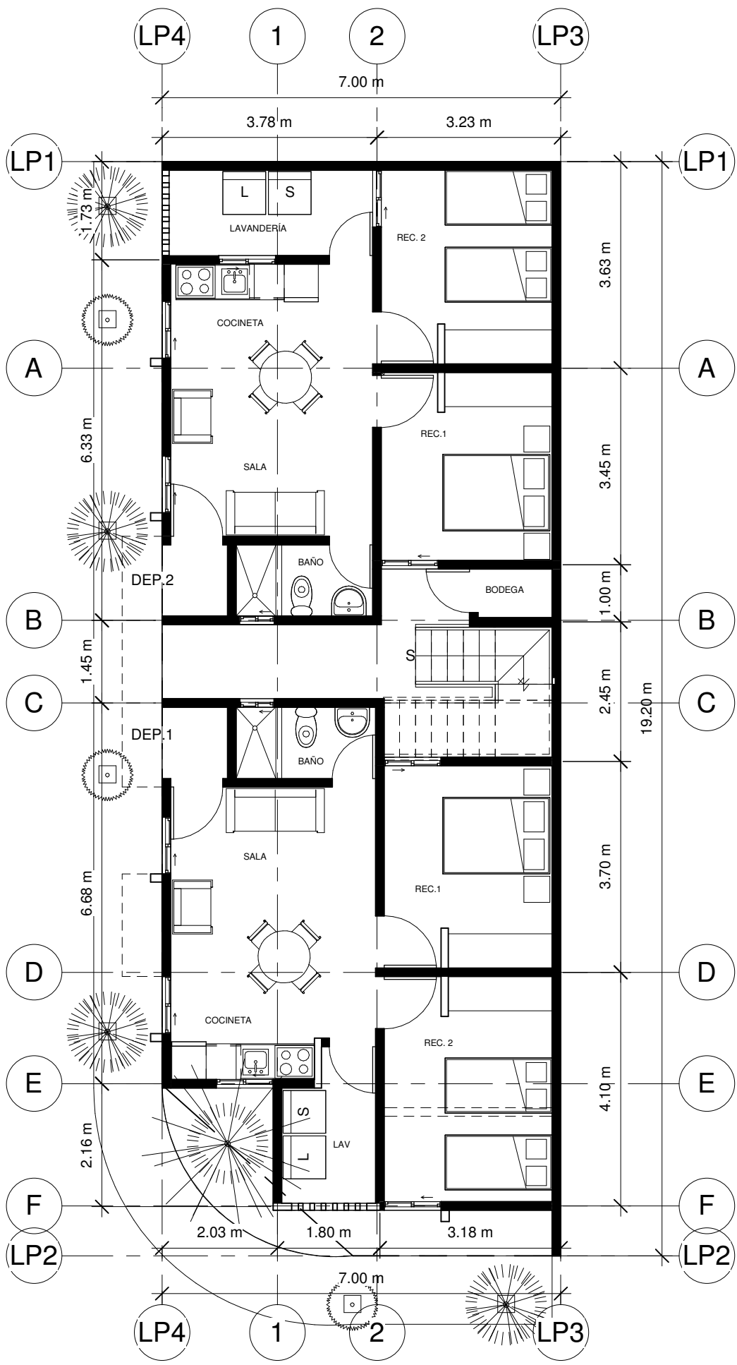
PLANTA BAJA
