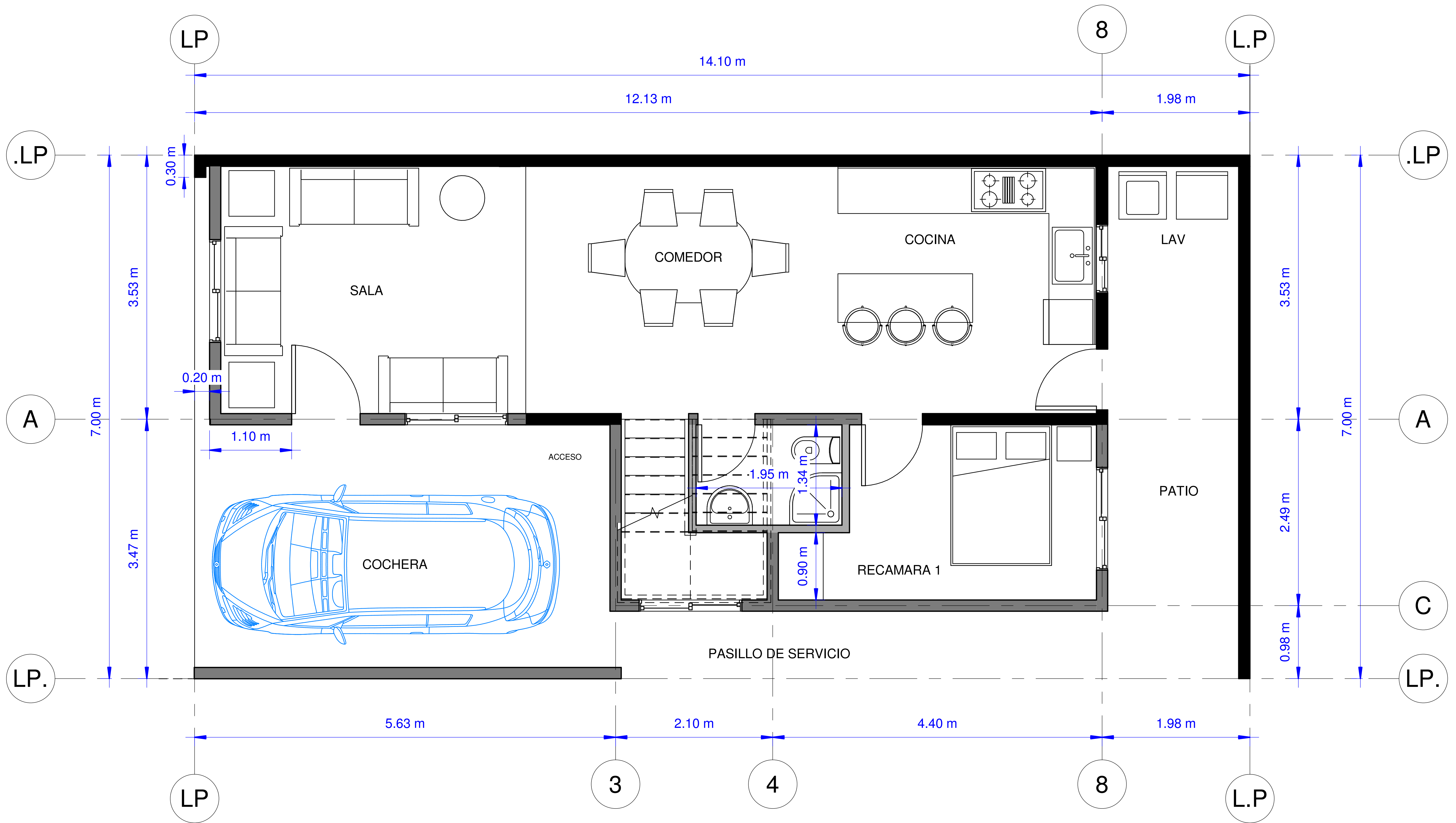
PLANTA ARQUITECTONICA BAJA
